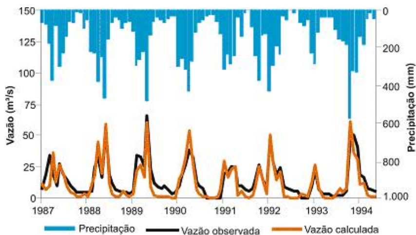
Figura 5. Hietograma médio observado e hidrogramas observados e calculados para o posto Pirapama durante a calibração do modelo.
